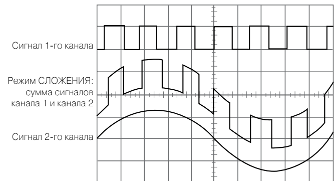
Рис. 37. Сложение сигналов
