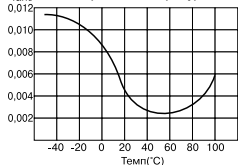
Зависимость тангенса угла потерь от температуры
