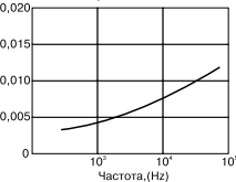
Зависимость тангенса угла потерь от частоты
